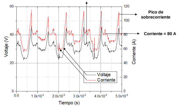
Figura 7 Voltaje y corriente durante la descarga de arco en condiciones controladas.
